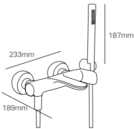
Miscelatore vasca esterno con set doccia Exposed bath mixer with shower set
