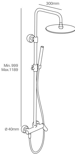
Miscelatore doccia esterno con colonna doccia soffione e doccetta Shower column with showerhead and shower set
