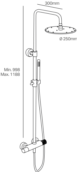
Miscelatore doccia esterno con colonna doccia soffione e doccetta Shower column with showerhead and shower set
