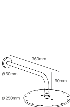
Soffione con braccio Shower head with arm
