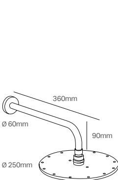
Soffione con braccio Shower head with arm
